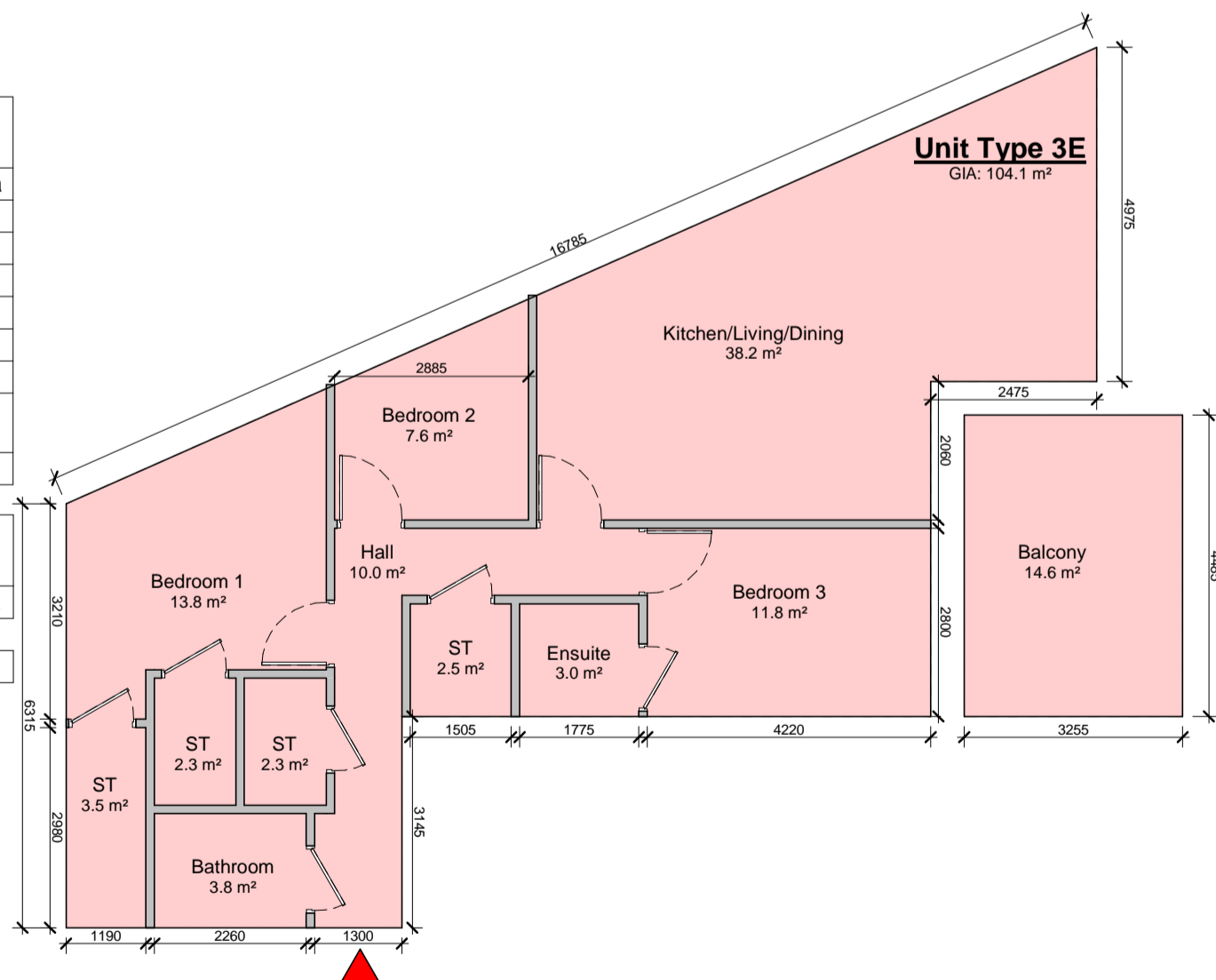
5 Apartment Type 3E 1 : 100
