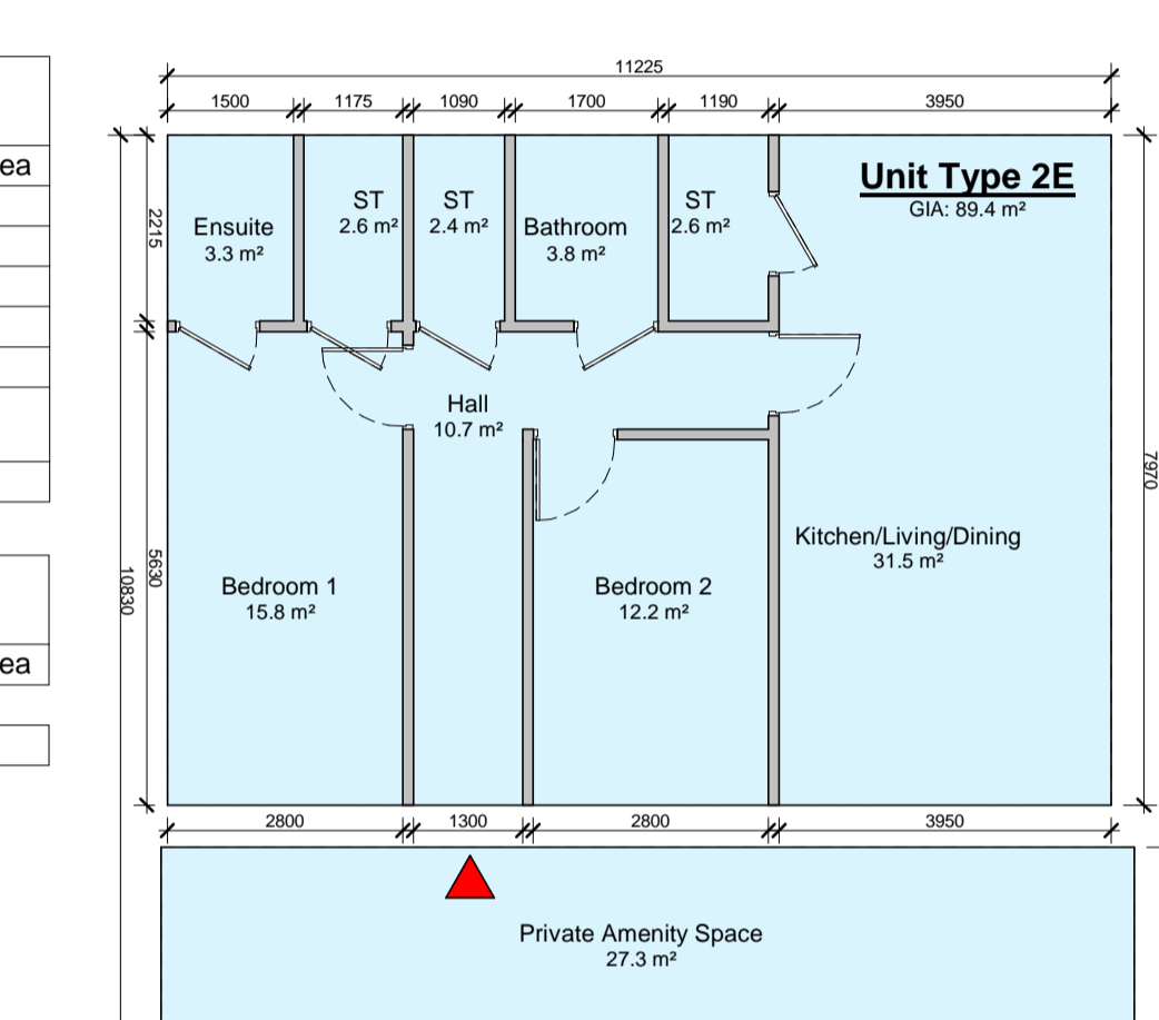
5 Apartment Type 2E 1 : 100
